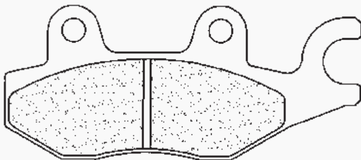
Dim. / Size 96.6 mm 42 mm 8 mm
