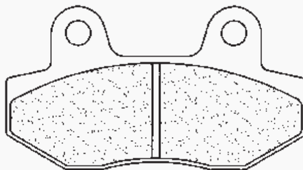
Dim. / Size 77 mm 42 mm 8 mm
